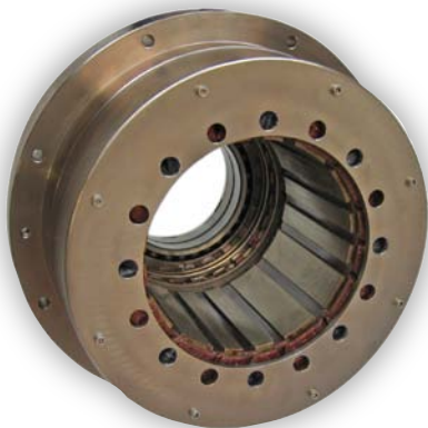
ラジアル軸受カートリッジ
