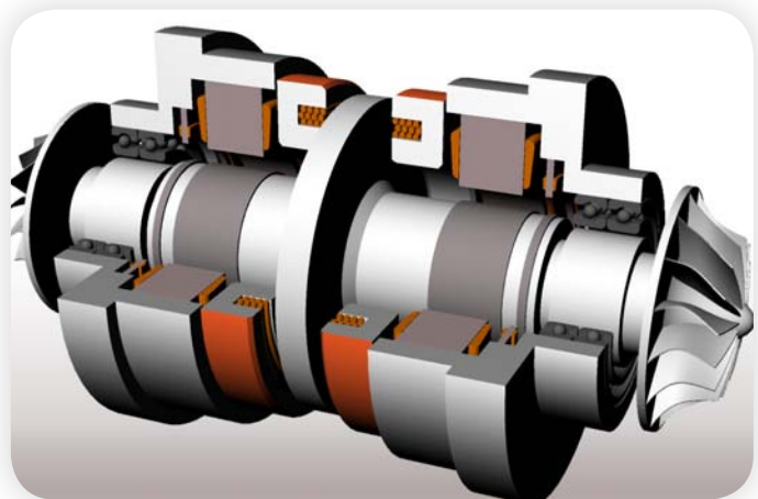
Vista geral do conjunto: 1 eixo + 2 cartuchos
